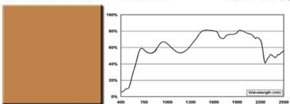
Brown 156 FeZnTi TSR 47%
