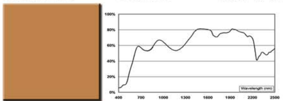
Yellow 10C242 CrSbTi TSR 66 %
