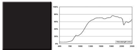
Black 411 A FeCr TSR 25%
