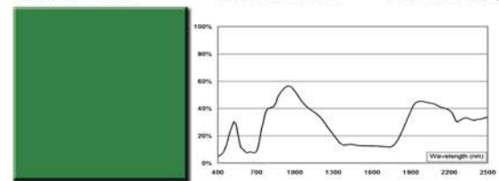
Green 410 CoCrZnTi TSR 25%
